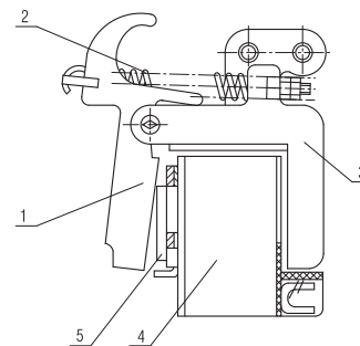
1 - якорь; 2 - пружина; 3 - ярмо; 4 - катушка; 5 - сердечник. Рисунок 9 - Расцепитель нулевого напряжения
